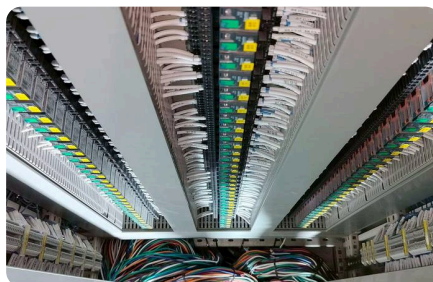
เข้าสายเทอร์มินอล
