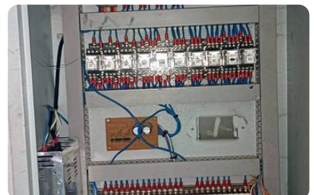
ตู้ควบคุมลิฟต์บรรทุก
